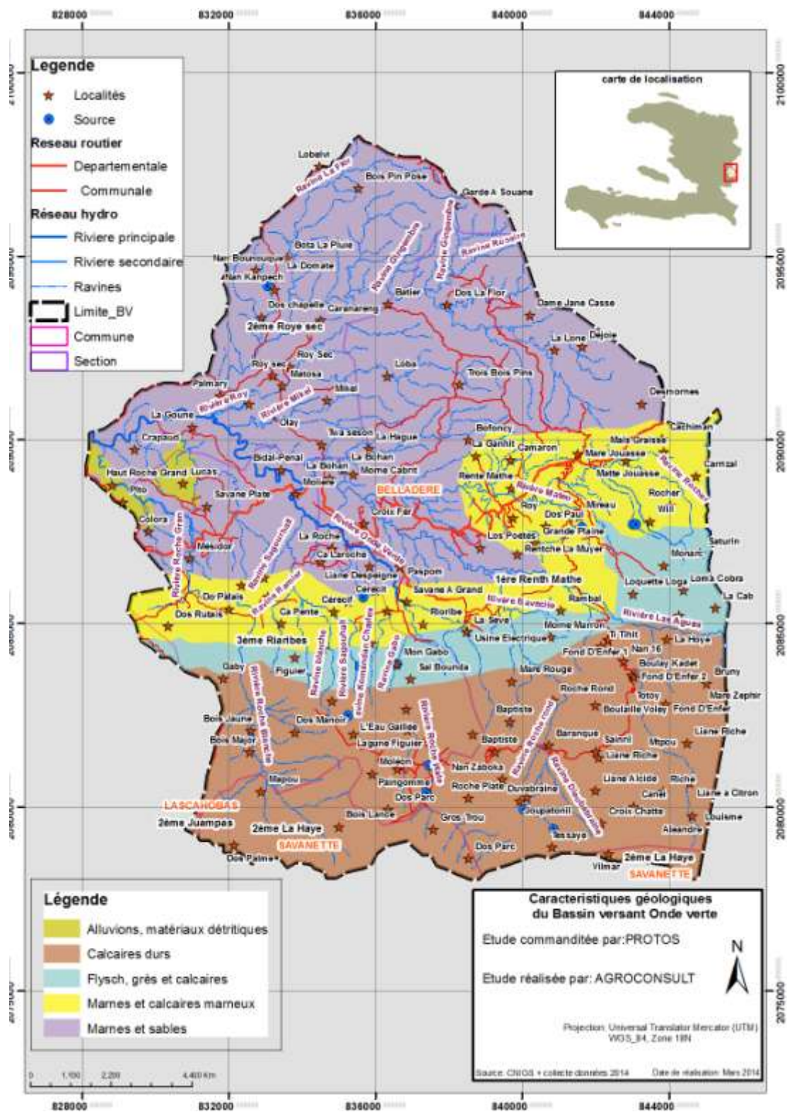
Carte 5. Caractéristiques géologiques du bassin versant Onde Verte
