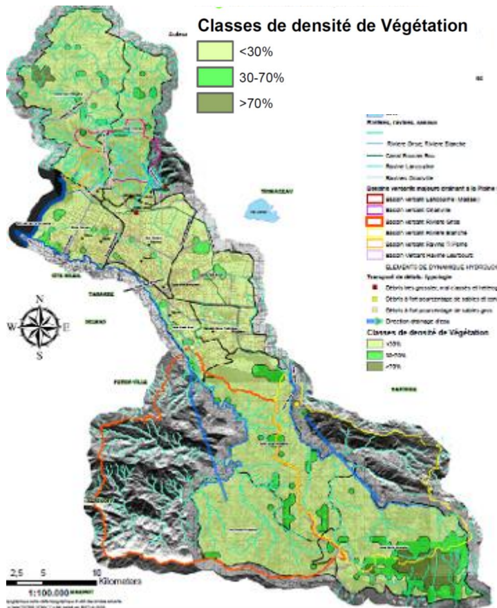
FIG. 47: Carte de végétation avec la délimitation des bassins versants et l'indication des directions de drainage superficiel des eaux du bassin.
