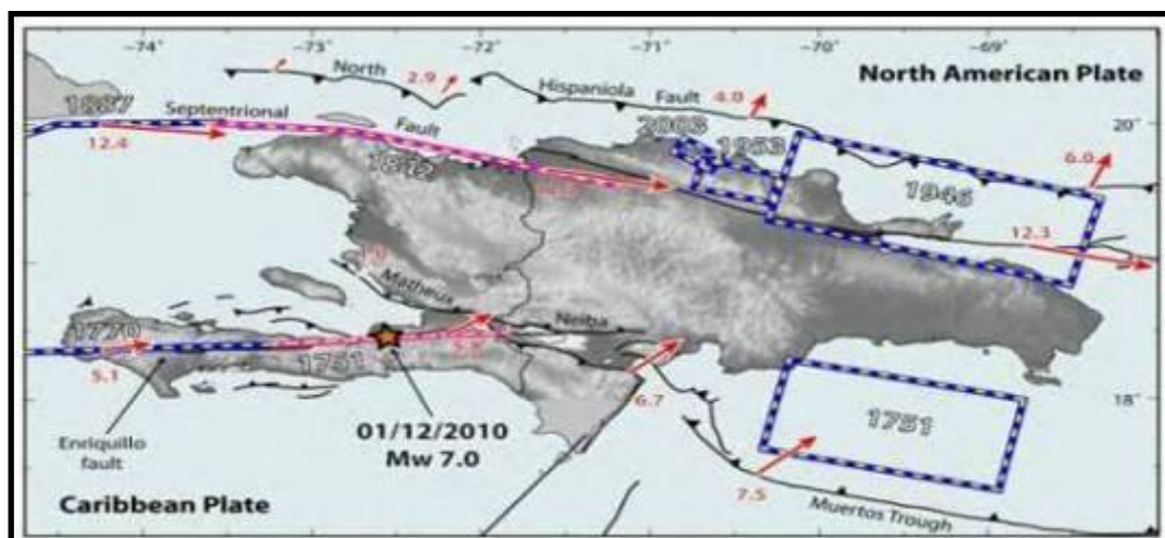
FIG.. 10 Les études de Calais et Hasse en 2010, avec la mise en place de points GPS mettent en évidence l'activité sismique de la Chaîne des Matheux avec une vitesse du mouvement de 1mm/a.
