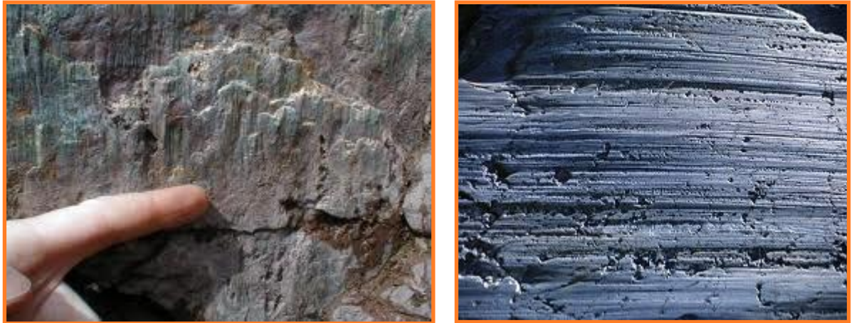
FIG. 18 : Éléments qui peuvent être présentés dans les plans de failles et qui montrent le mouvement de faille.
