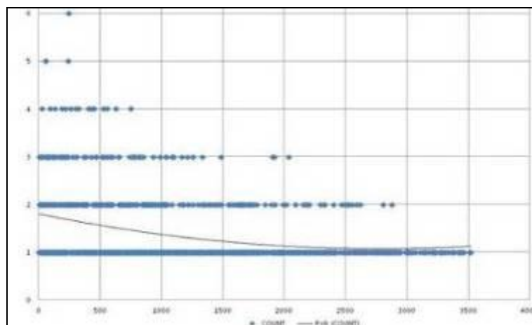
Fig. 35: Graphique pour la détermination d'indice d'influence des failles aux glissements et les distances.
