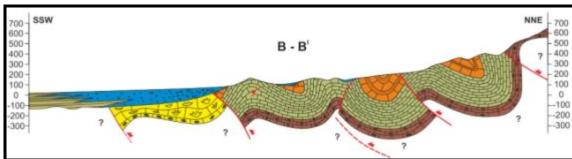
Figura 1 Profil géologique dans la zone de Canaan, Onanville qui montre les plis* tectoniques* de direction SSO.
