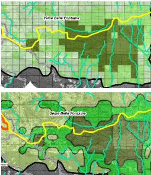
FIG. 45 : Élaboration de la carte de densité de végétation à travers les résultats de la photo-interprétation de la grille (en haut) et donc transformation en données continues (en bas).
