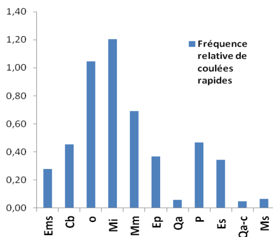
Fréquence relative de coulées rapides par lithologie
