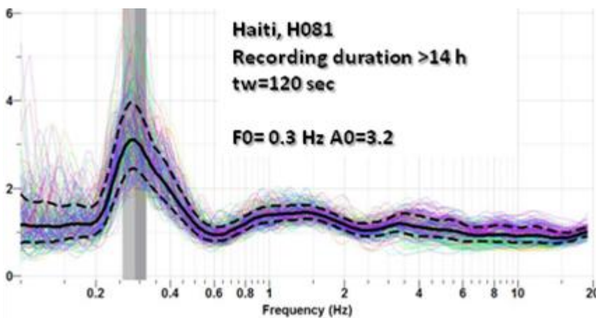
FIG. 23 : Exemple de courbe HV d'un test à longue durée (14 heures). Le point de mesure, comme pour la majorité de la plaine étudiée, est caractérisé par de possibles phénomènes de résonance à fréquences plus basses que 0.5 Hz.
