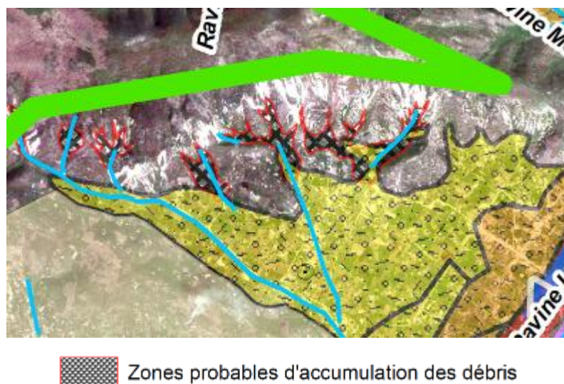
FIG. 60: Symbole des zones d'accumulation des débris.
