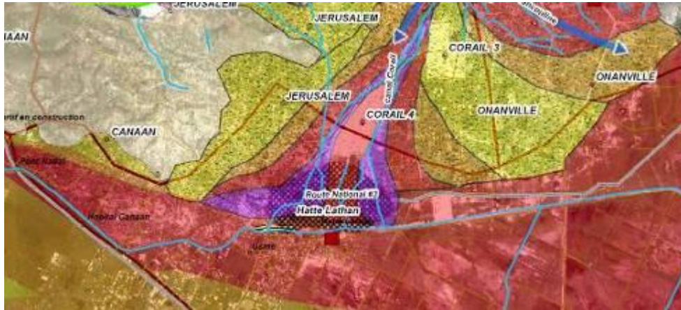
FIG, 65 : Zones à aléas plus forts causés par la ravine Lancouline.
