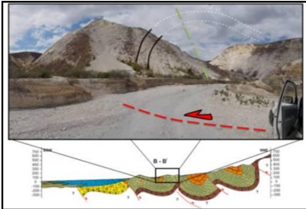
Figure 9 Affleurement du pli compressif de l'hanging wall* de la faille inverse de chevauchement de la ravine Lan Couline.
