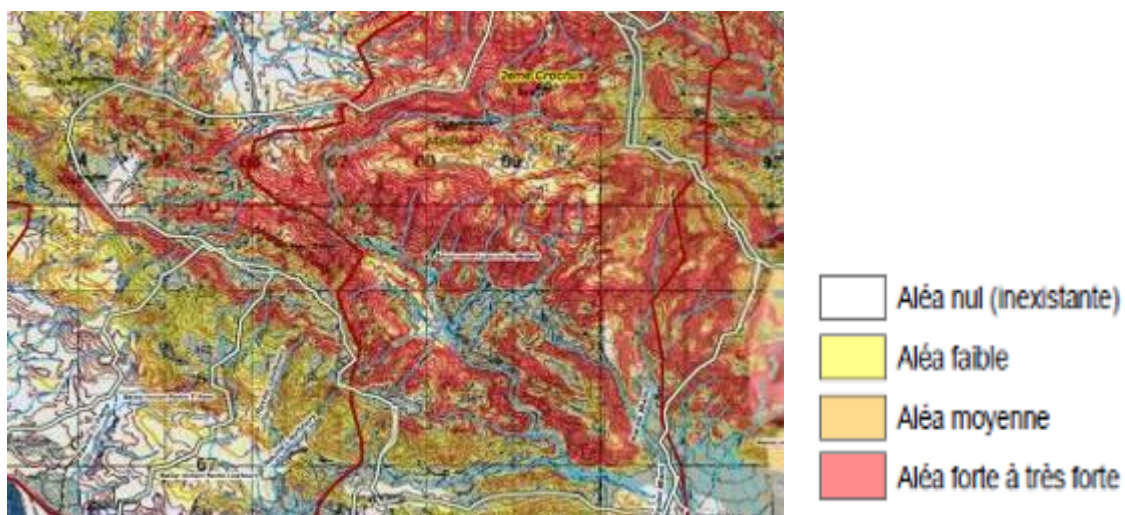
FIG. 38: Aléas de menace de détachement des glissements en débris dans le bassin versant de la ravine Lancoulaine.
