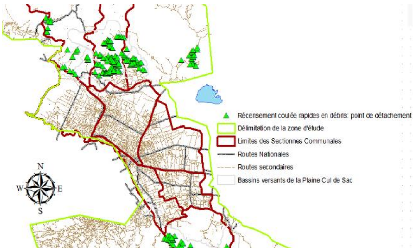
FIG. 31 Recensement des glissements en débris dans les dix sectionnes de Croix des Bouquets.
