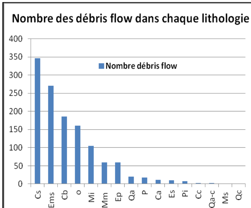
FIG. 32: Fréquence absolue des coulées rapides recensées dans chaque lithologie.
