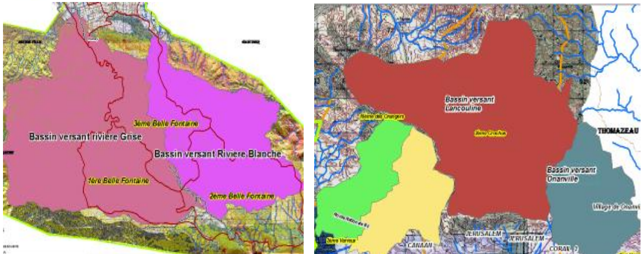
FIG. 3: Bassins versants majeurs drainant à la Plaine Cul de Sac.
