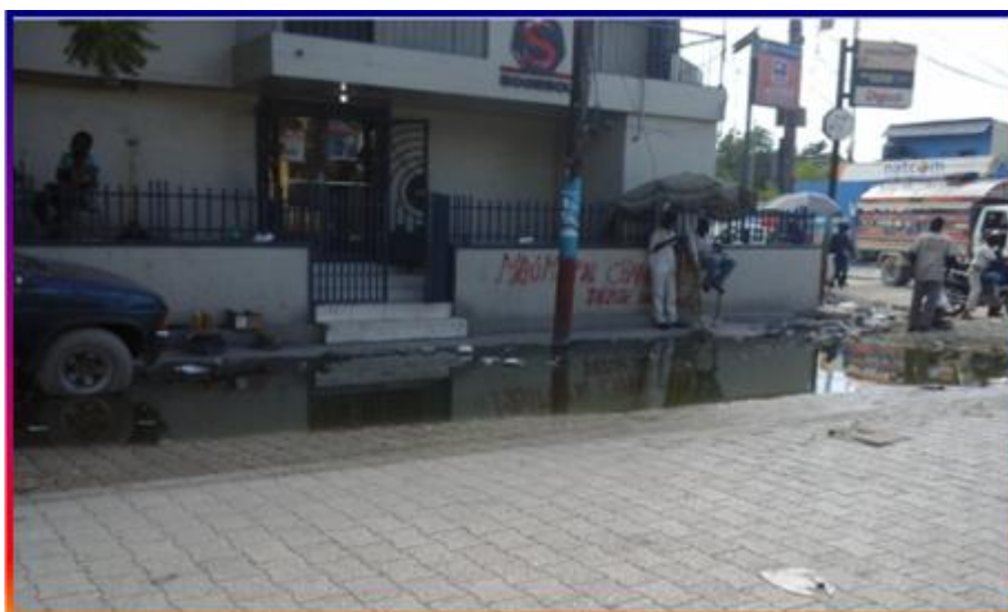
FIG. 56: Zones de ruissellement urbain (2 ème Varreux).
