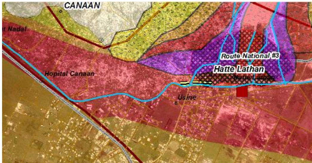
FIG, 70 La carte de menace hydrologique qui montre les habitations de l'Usine et de l'hôpital de Canaan dans la zone des aléas forts.
