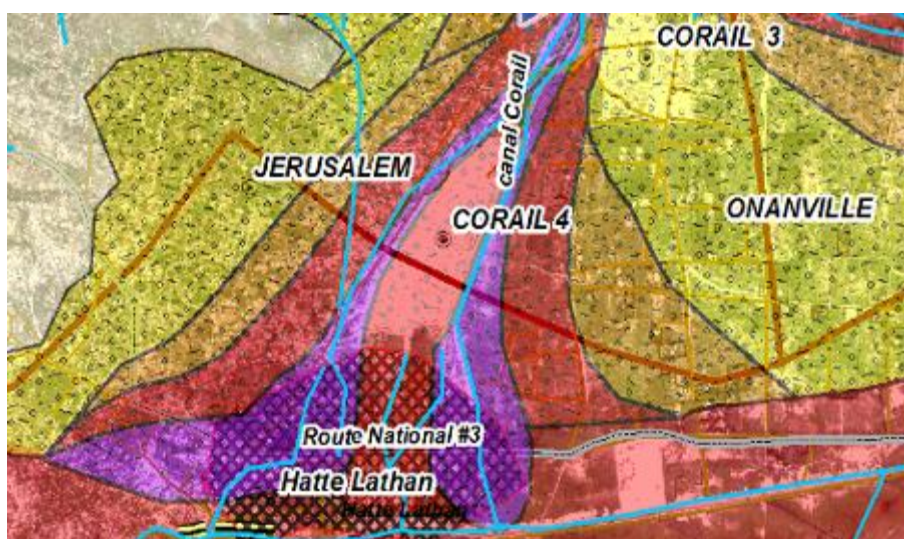
FIG, 71 En haut maisons construites à coté de la ravine Lancouline, dans la partie plus au Nord près du Camp Corail 3. En bas les aléas forts et très forts dans la zone du Camp Corail 4.
