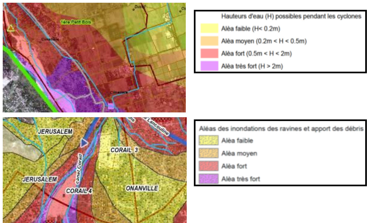
FIG. 49 : Symbololes des aléas hydrologiques: en haut les aléas de la Plaine Cul de Sac (eaux des inondations des rivières Grise, Blanche, canal Broucanbrou et canaux urbains); en bas les aléas des ravines de Onanville, Jérusalem et Canaan (eaux et débris des ravines).
