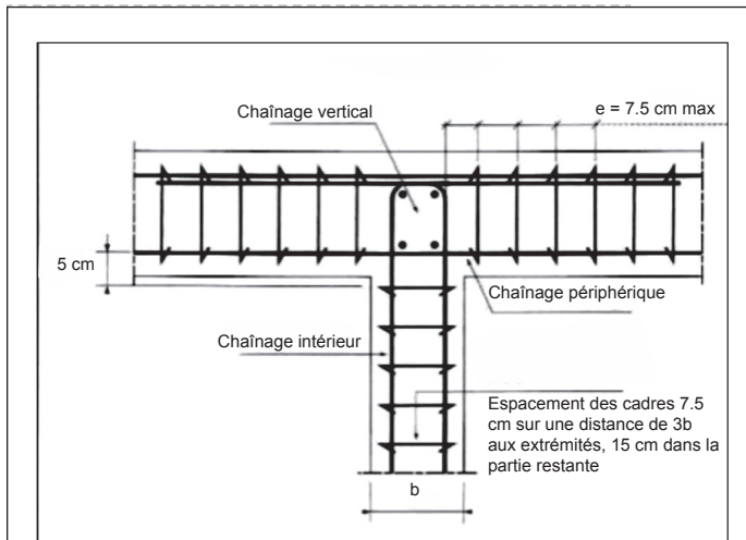
Dessin 52 : Exemple de liaison entre chaînages en partie courante
