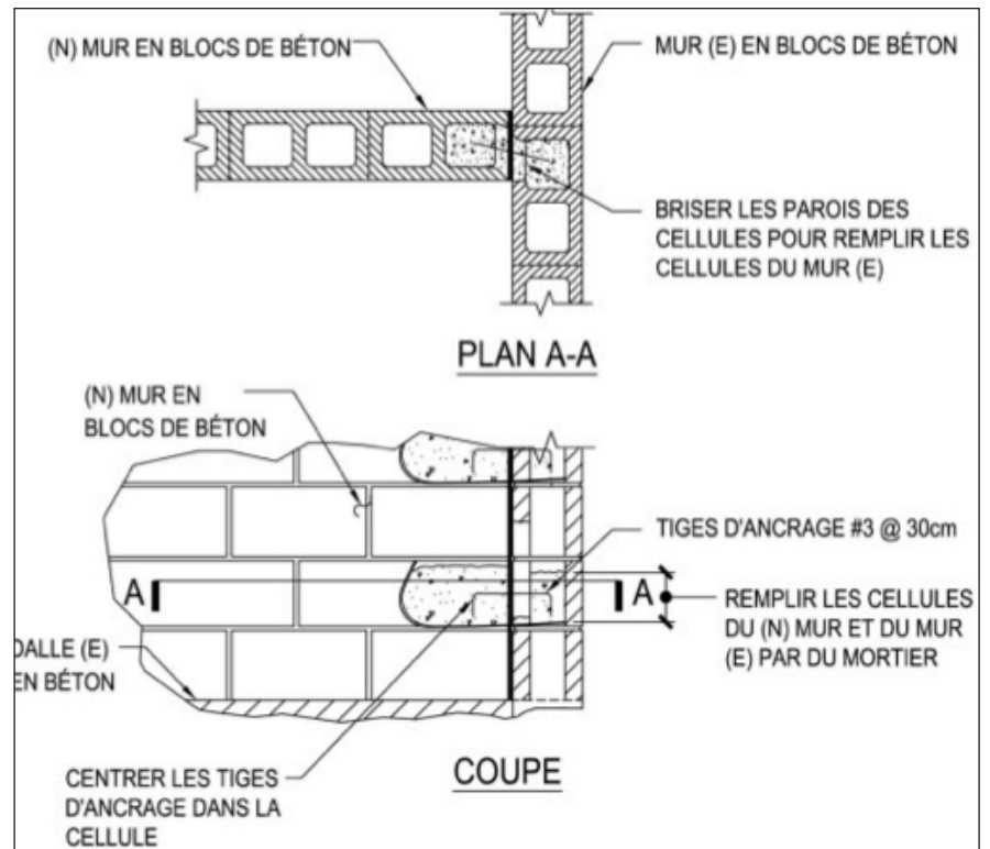
Dessin 46 : Connexions renforcées aux angles
