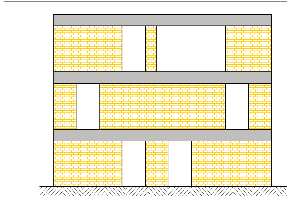
Dessin 18 : Ouvertures non superposées
