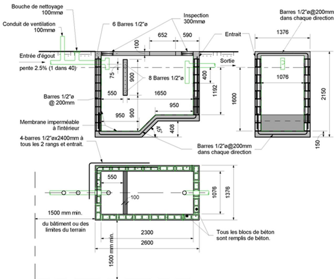
Figure 1.5.10.3.b - Fosse septique de 3 200 litres – 8 personnes maximum
