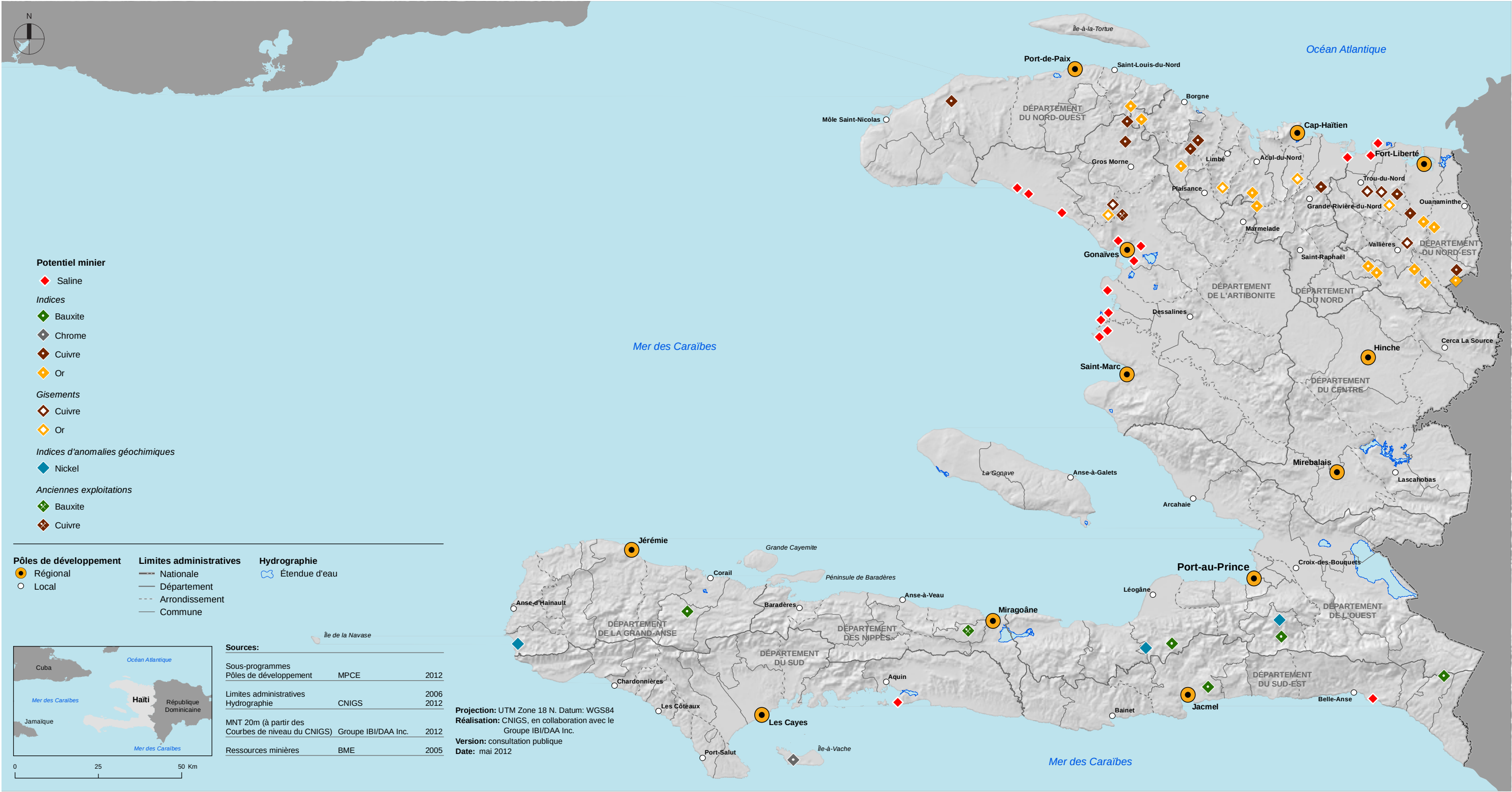
Carte 19 : CARTE DES POTENTIELS MINIERS
