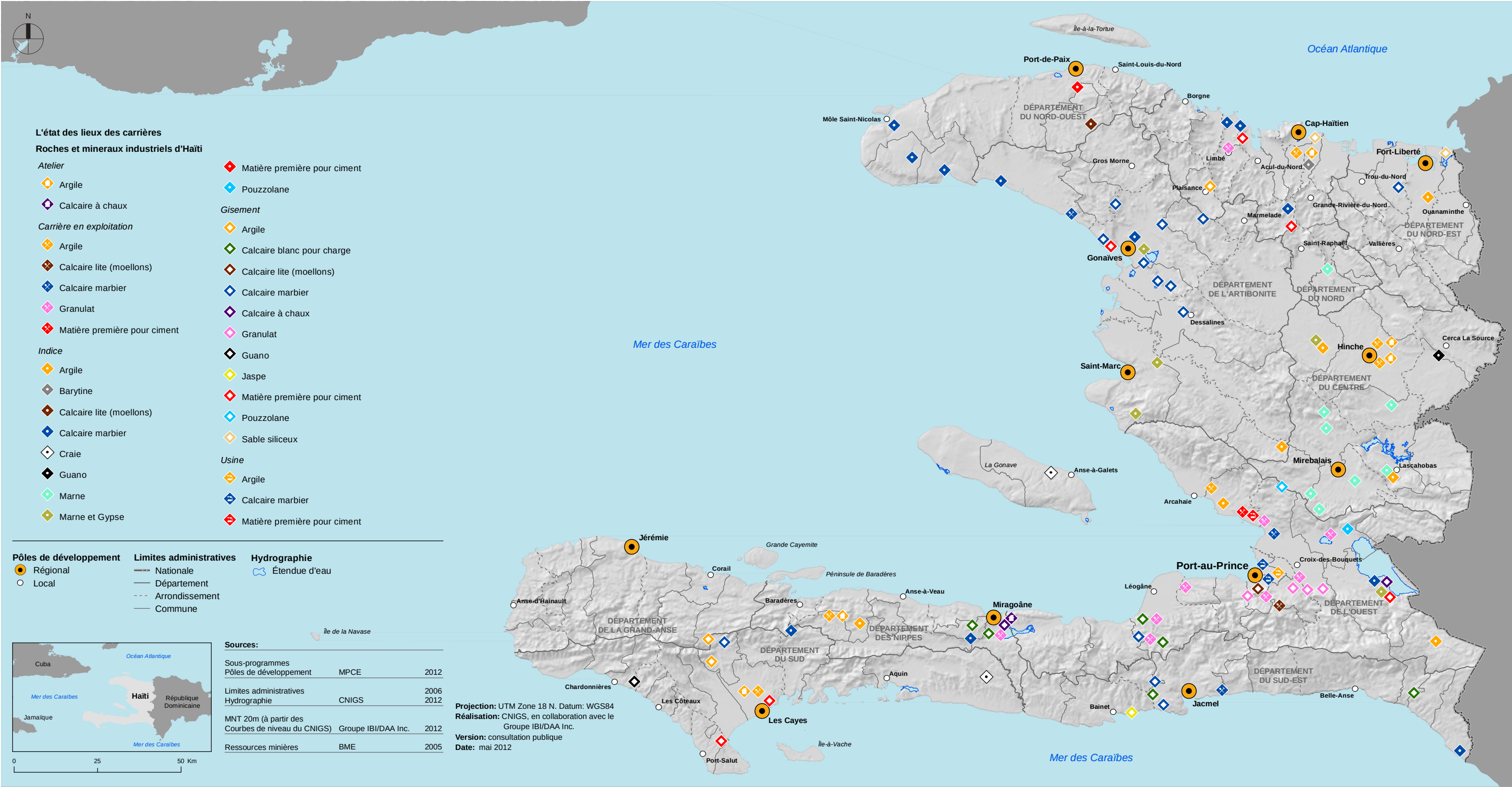
Carte 20 : CARTE DE L'ÉTAT DES LIEUX DES CARRIÈRES
