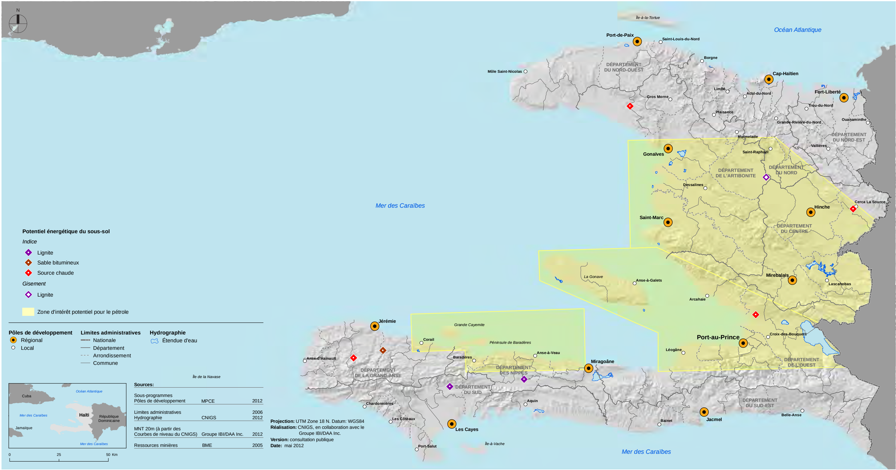
Carte 21 : CARTE DU POTENTIEL ÉNERGÉTIQUE DU SOUS-SOL
