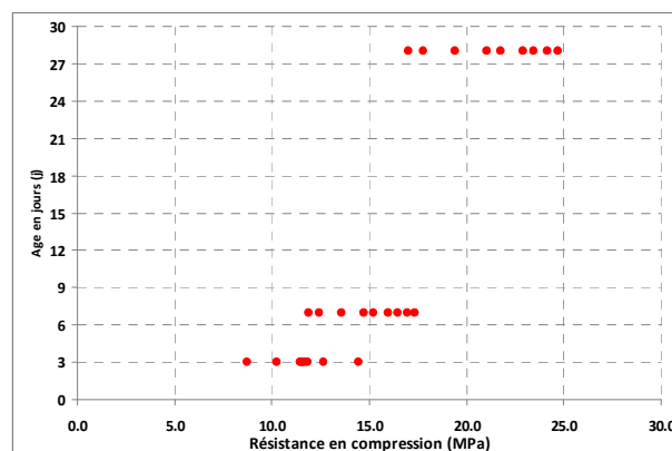
Figure 4. Résistances en compression des matériaux en fonction des âges (3, 7 et 28 jours)
