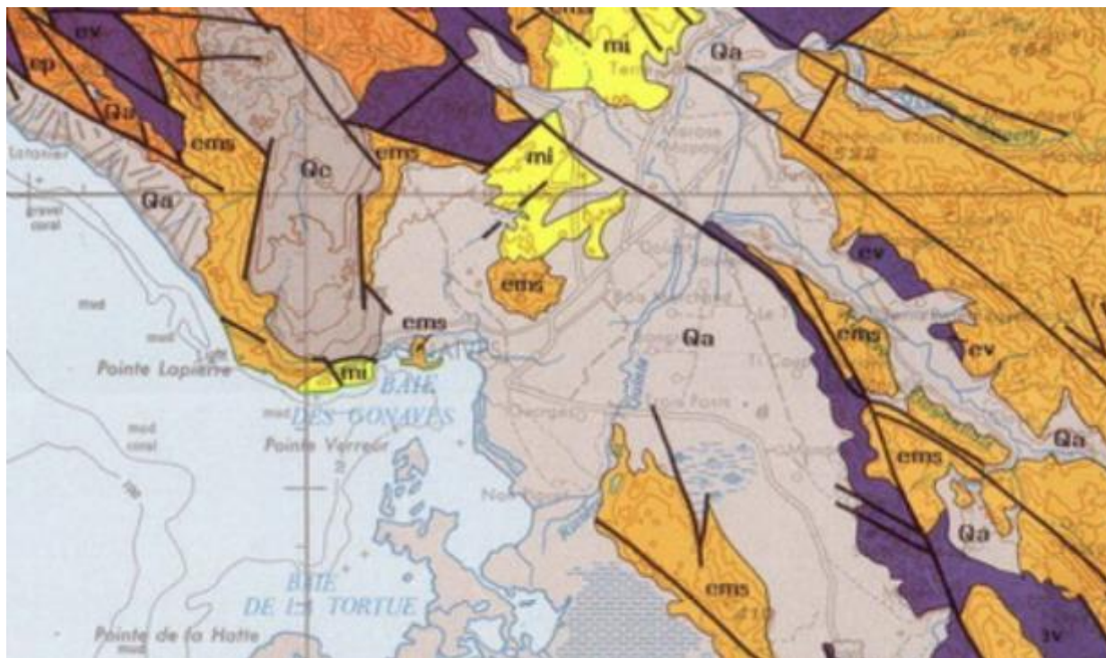
Figure 4-2 : Carte géologique de la Baie de Gonaïves (carte géologique d'Haïti au 1/250000, feuille Nord-Est, 1987)
