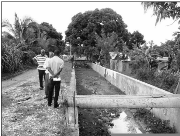
Mur de tête à l'entrée du Dalot 1
