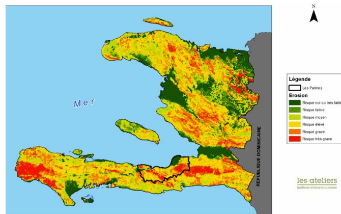
les zones d'érosion source: DATIP
