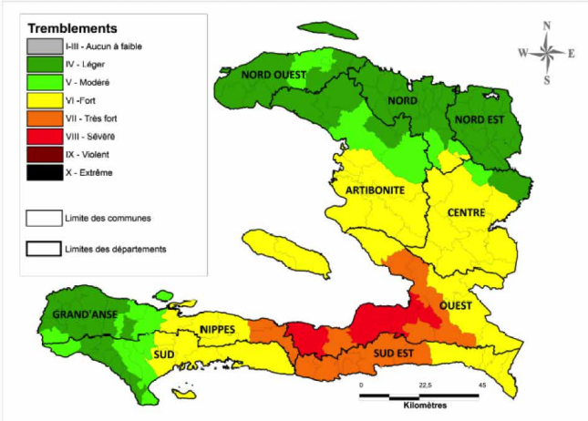
Carte d'intensité du séisme selon l'indice PGA^2 , échelle de Mercalli
