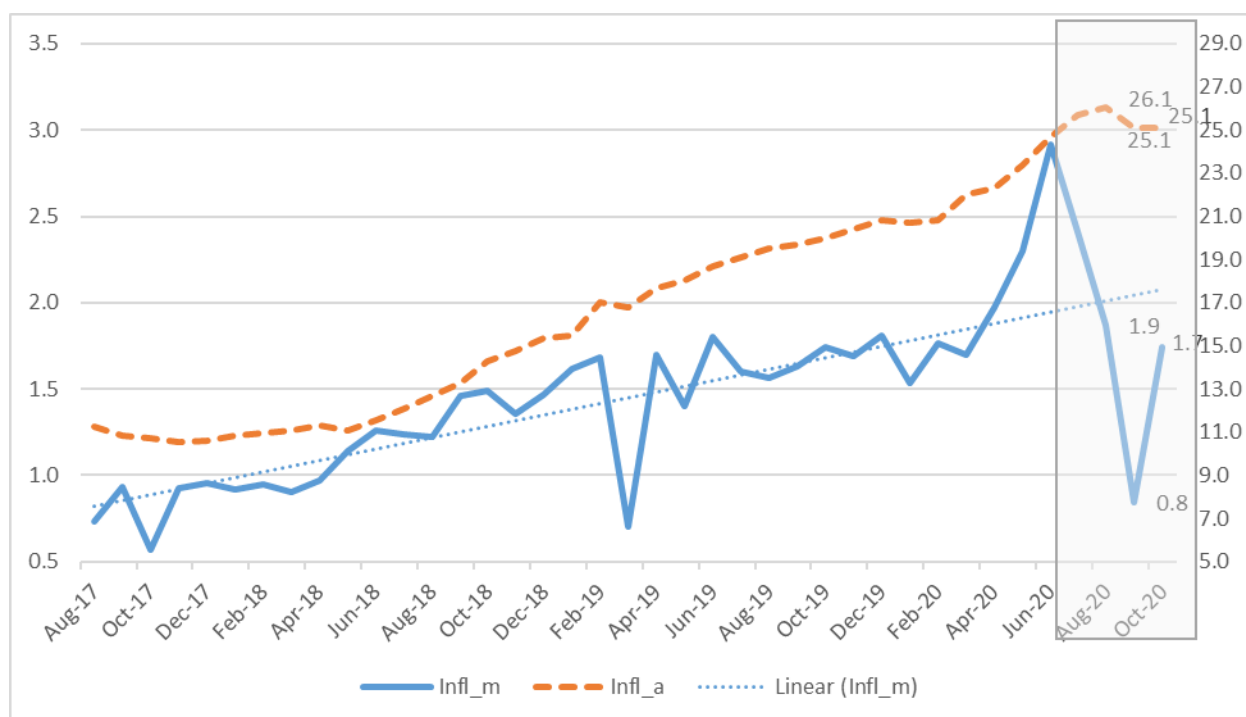
Graphique 3 Prévisions de l'inflation en variation mensuelle et en glissement annuel sur trois mois (en %, à partir du mois d'août 2020)
